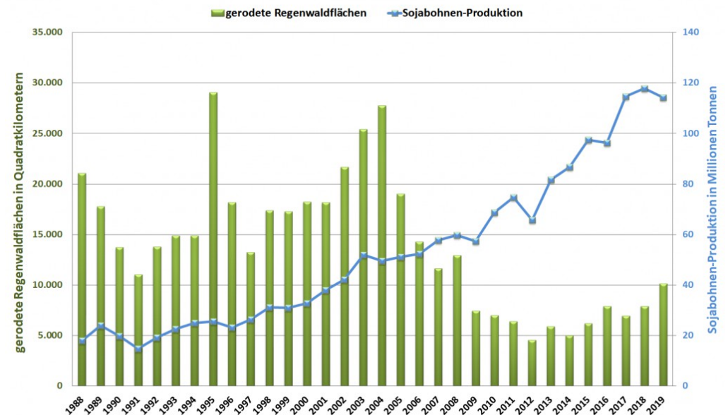
Regenwaldrodungen und Sojabohnen-Produktion in Brasilien (1988 - 2019)
